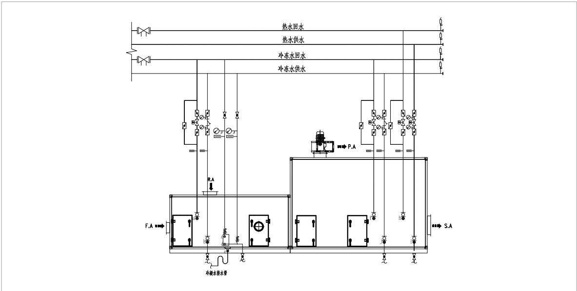
（接管示意图）
