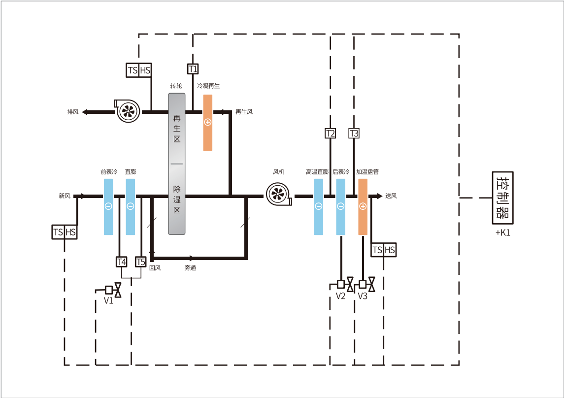
附：系统用控制图
