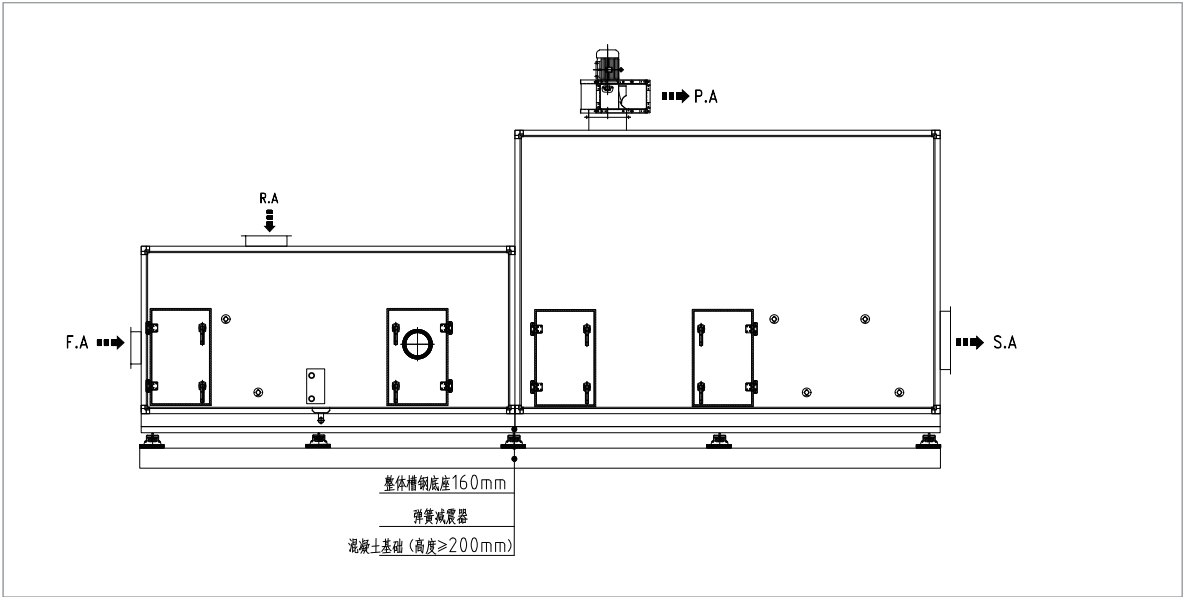
（机组安装基础示意图）
